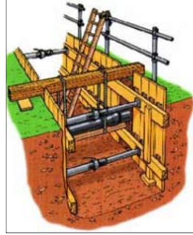
Şekil 5 – Hendek güvenlik önlemi
