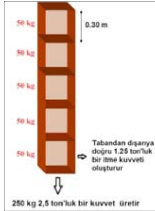
Şekil 2 – Toprağın oluşturduğu kuvvet
