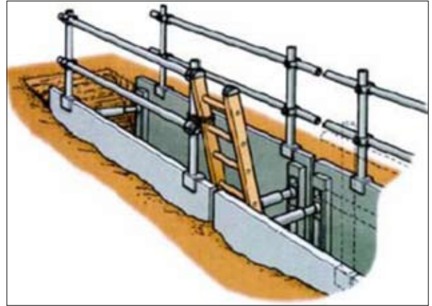
Şekil 6 – Hendek korkuluğu
