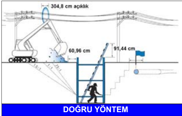
Şekil 4 – Kazı da iş makinasının doğru kullanımı (23)
